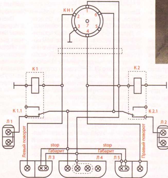
Рис. Принципиальная схема
