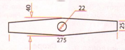
Рис 2 Чертеж ножа
